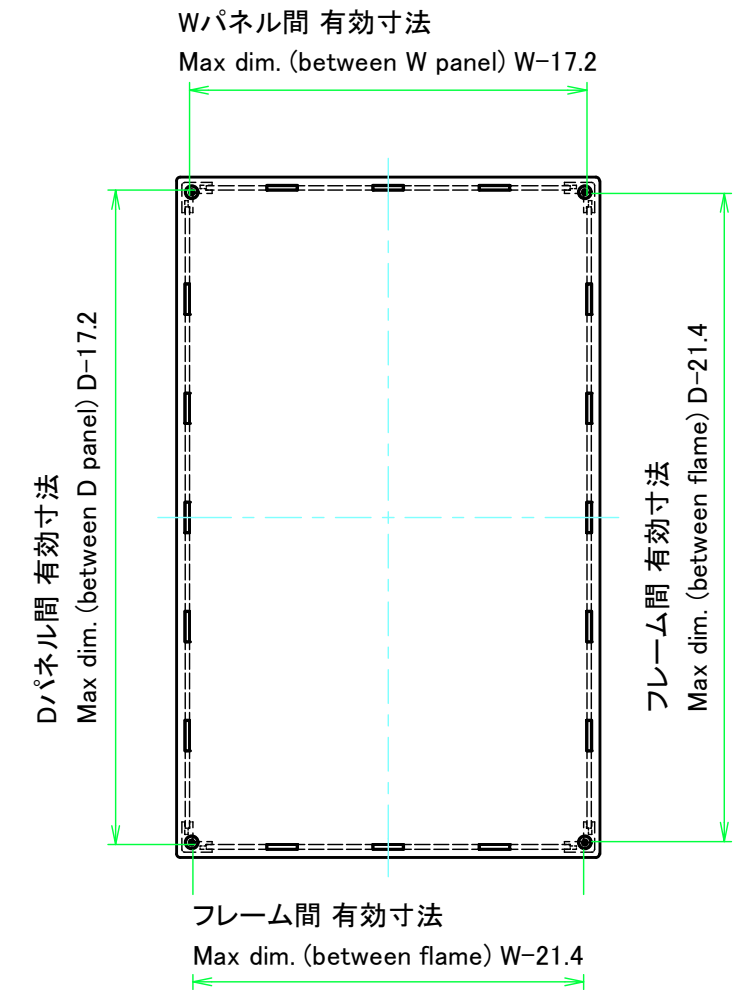
下カバー / Bottom cover
